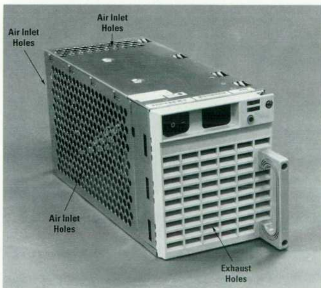
Fig. 8. Power supply module.
